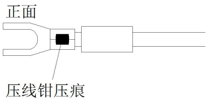
图 3.2.2 U 型冷压端子压线钳压痕示意图（以现场提供的 U 型冷压端子为准）
