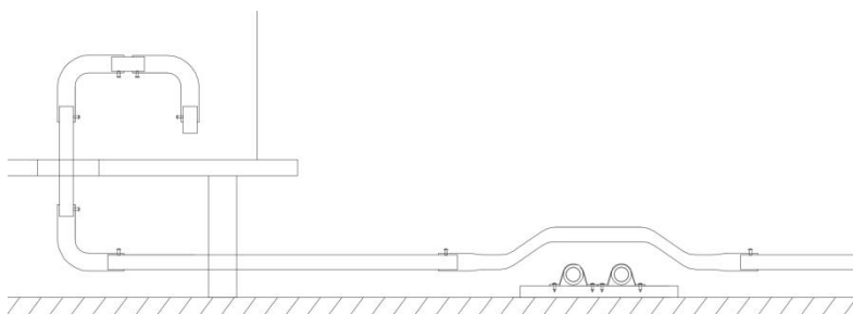
图 3.2.5 户外布管示例 1
