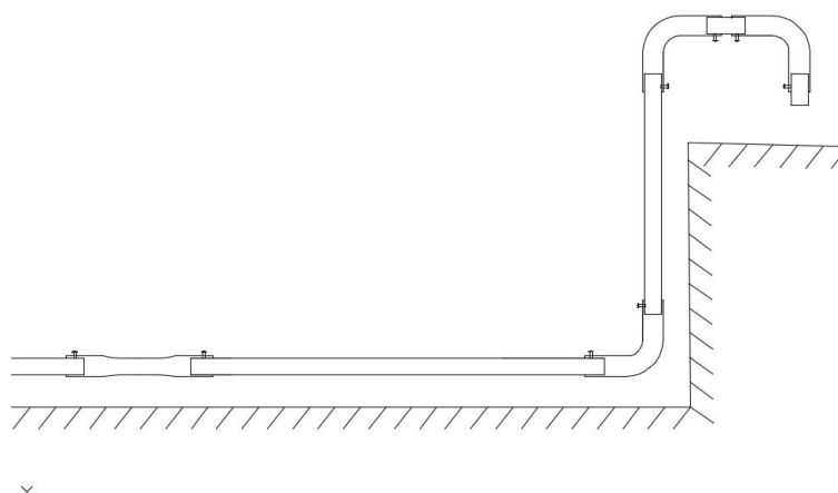
图 3.2.6 户外布管示例 2
